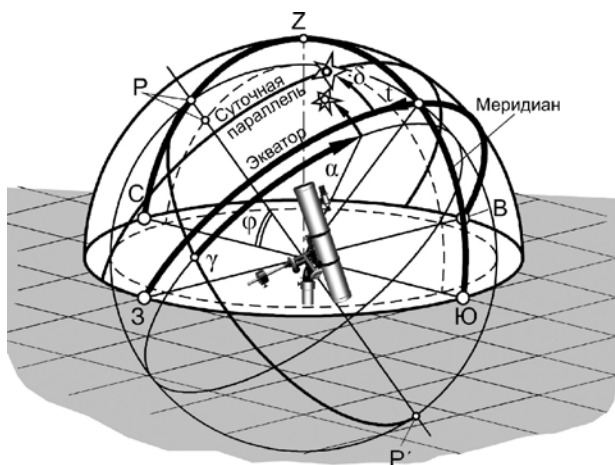
Рисунок 1 – Подвижная и неподвижная экваториальные системы координат
